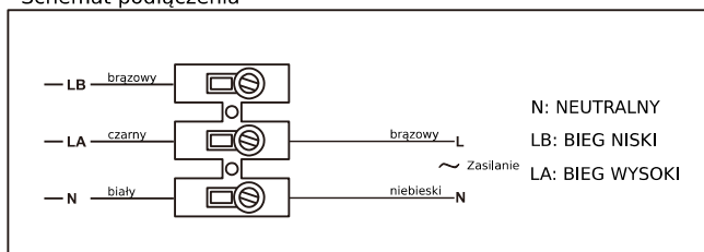
Schemat podłączenia z regulatorem obrotów
